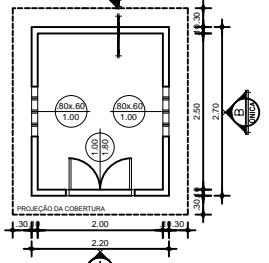
PLANTA BAIXA ESC. 1/50
