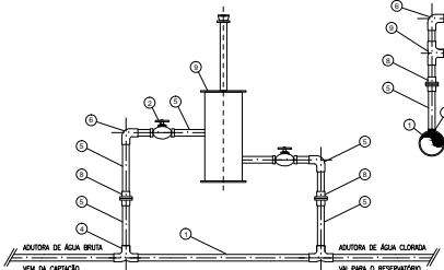
VISTA FRONTAL - Clorador de pastilha SEM ESCALA
