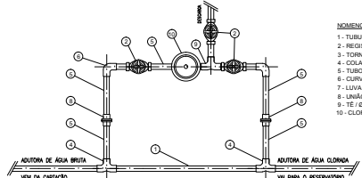
VISTA SUPERIOR Clorador de pastilha SEM ESCALA
