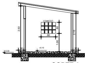
CORTE A ESC. 1/50
