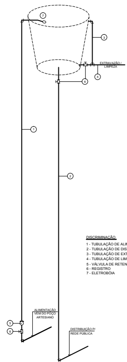
ESQUEMÁTICO DE RESERVATÓRIO ELEVADO ESC. 1/50
