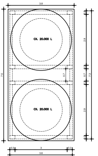
PLANTA BAIXA ESC. 1/50
