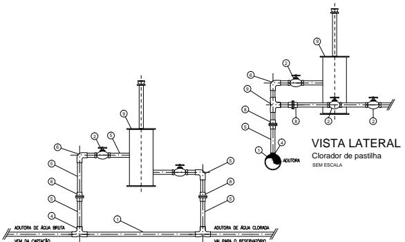
VISTA FRONTAL - Clorador de pastilha SEM ESCALA
