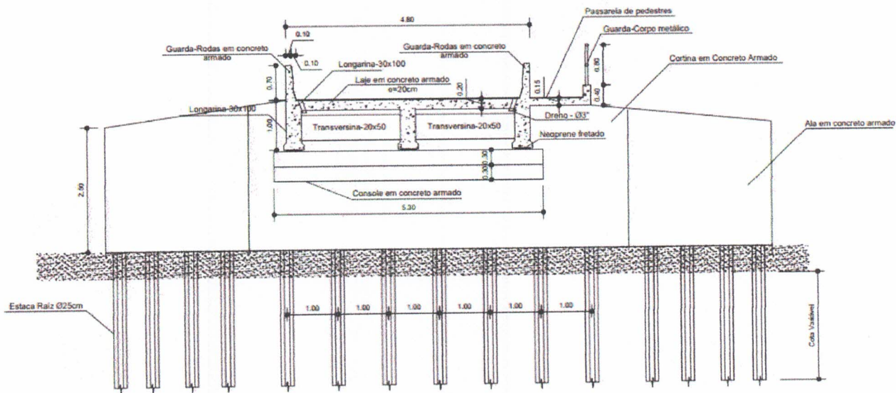
SEÇÃO-01 PONTE TV. SÃO JOAQUIM
