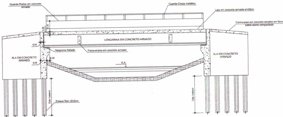
SEÇÃO-02 PONTE TV. SÃO JOAQUIM
