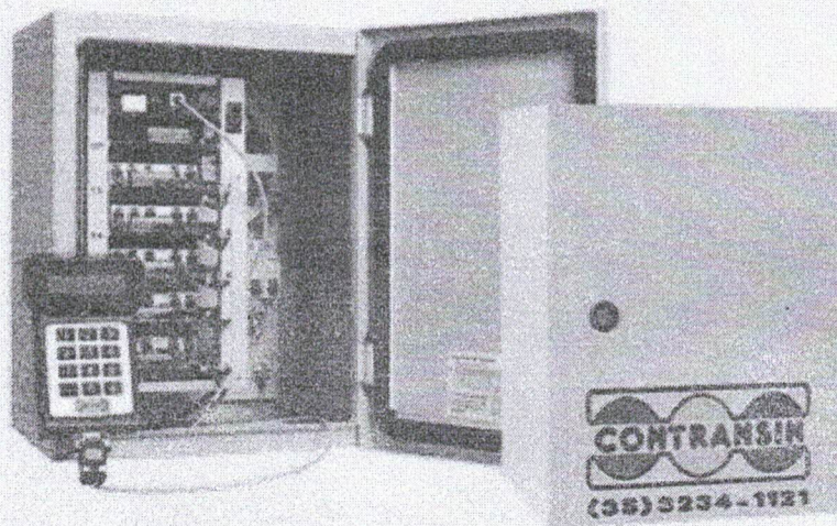
Controlador eletrônico de tráfego 2 fases.
